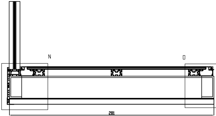
AlClad Decor SCALE 1:1
