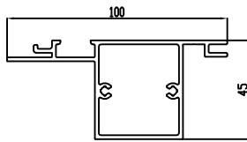
AlClad Decor SCALE 1:1
